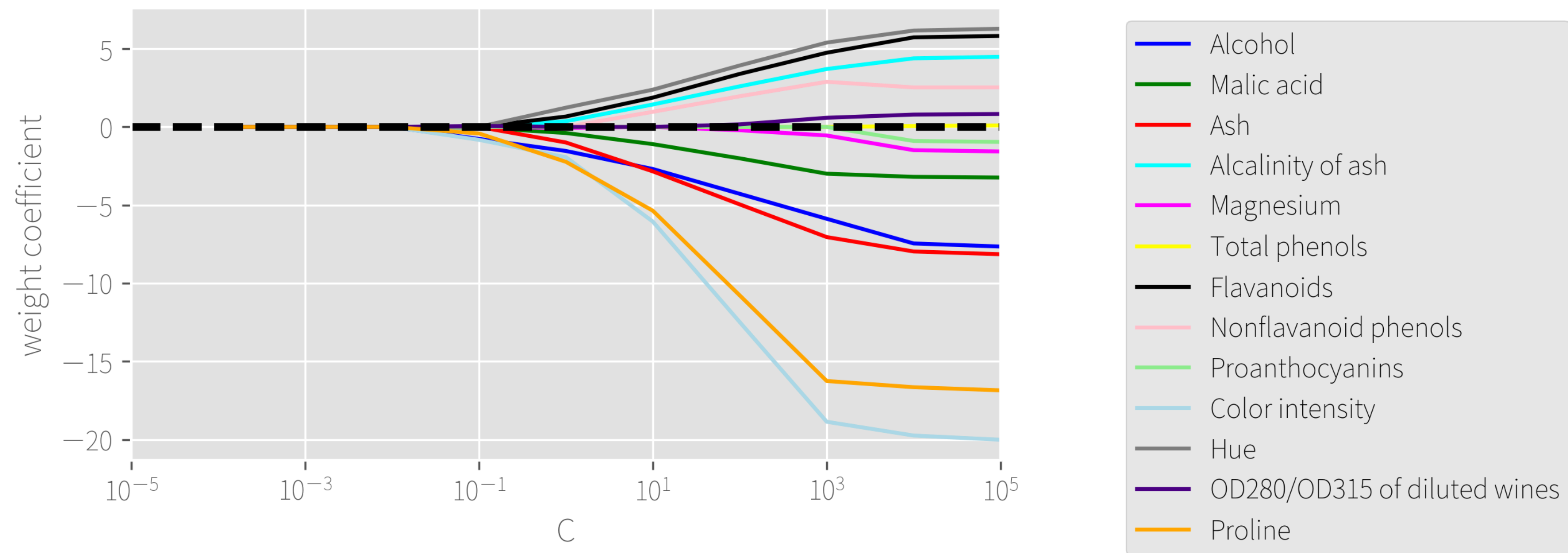
红酒分类正则化（ C 是正则化参数 \lambda 的逆，越小表示正则化强度越大）
